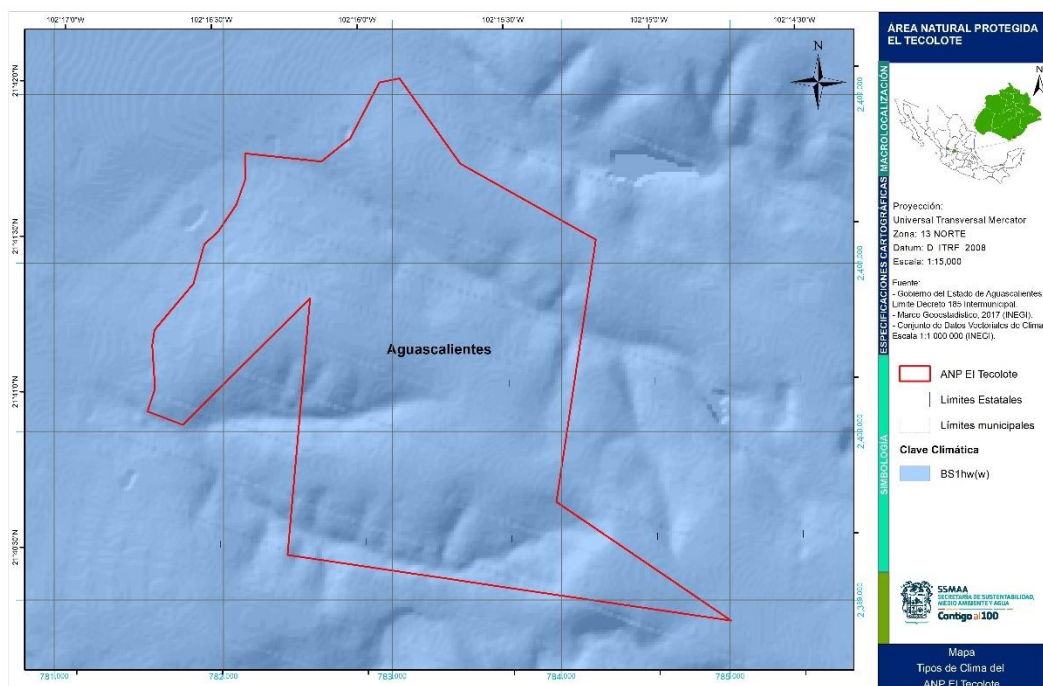
Figura 12. Mapa Tipos de Climas en el ANP El Tecolote
