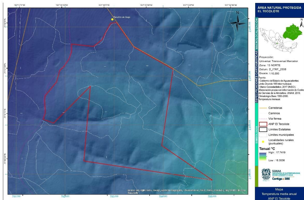
Figura 14. Mapa Temperaturas Media Anual en el ANP El Tecolote
