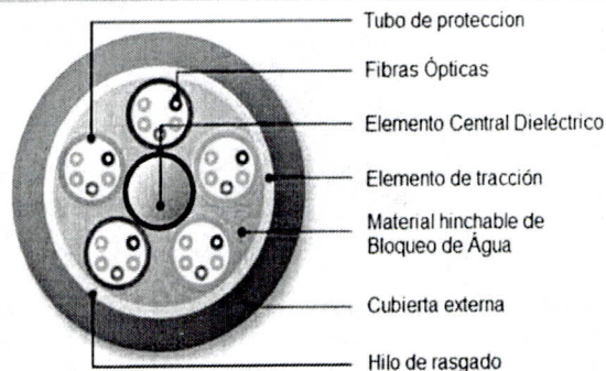
Sección Transversal
