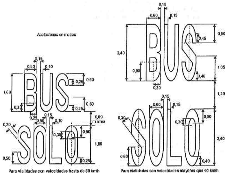
FIGURA 21.- Legenda SOLO BUS
