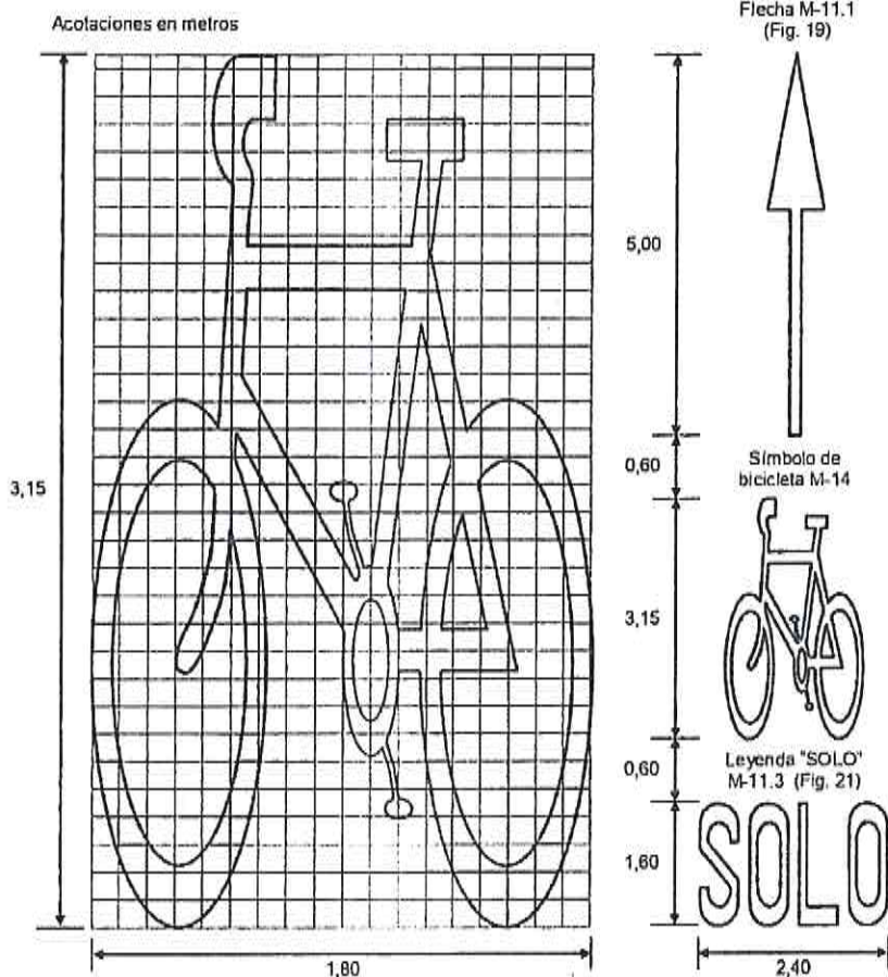
FIGURA 25.- Marcas para identificar ciclovías
