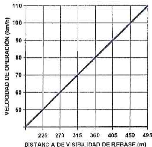
FIGURA 28.- Distancia de visibilidad de rebase
