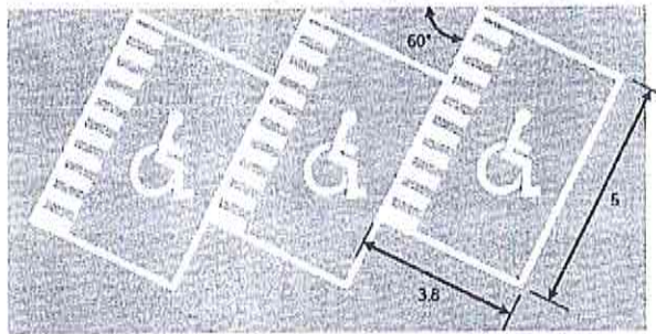
FIGURA 18.- Marcas de estacionamiento para vehículos de personas con discapacidad
