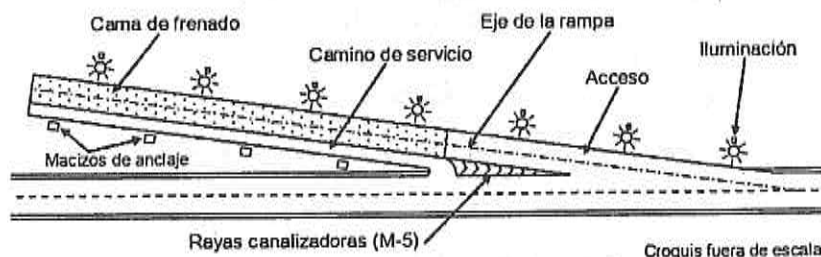
FIGURA 12.- Rampa de emergencia para frenado
