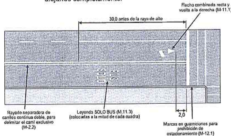
FIGURA 10.- Marcas para delimitar un carril exclusivo
