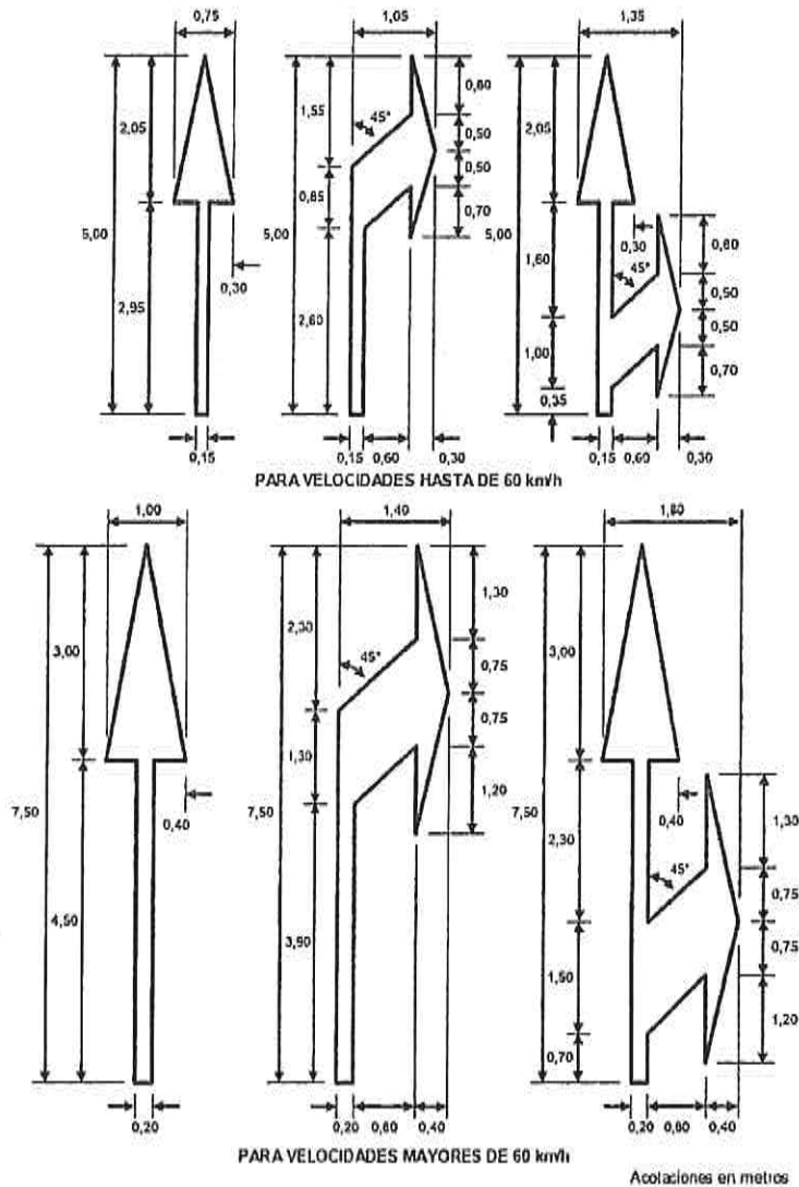
FIGURA 19.- Flechas de dirección para carriles
