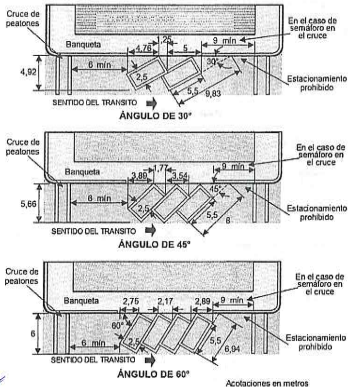
FIGURA 17.- Marcas para estacionamiento en batería
