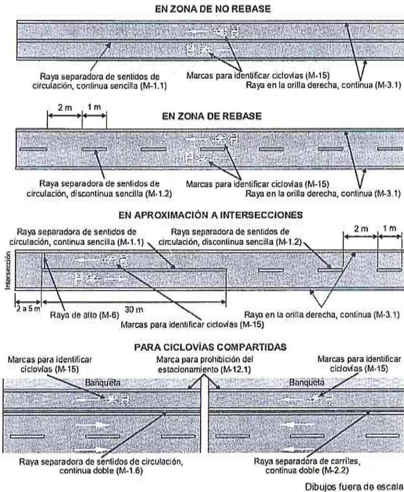
FIGURA 4.- Marcas en el pavimento para ciclovías
