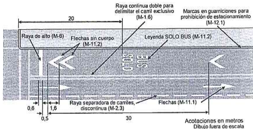
FIGURA 7.- Marcas para delimitar un carril en contrasentido
