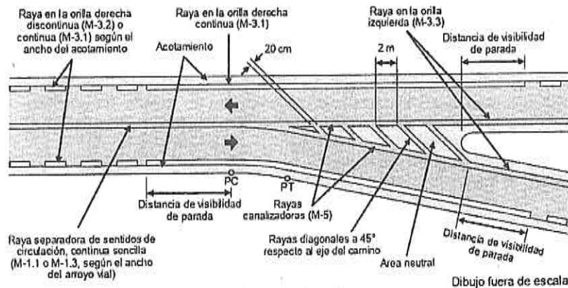
FIGURA 11.- Rayas en la orilla derecha y rayas canalizadoras
