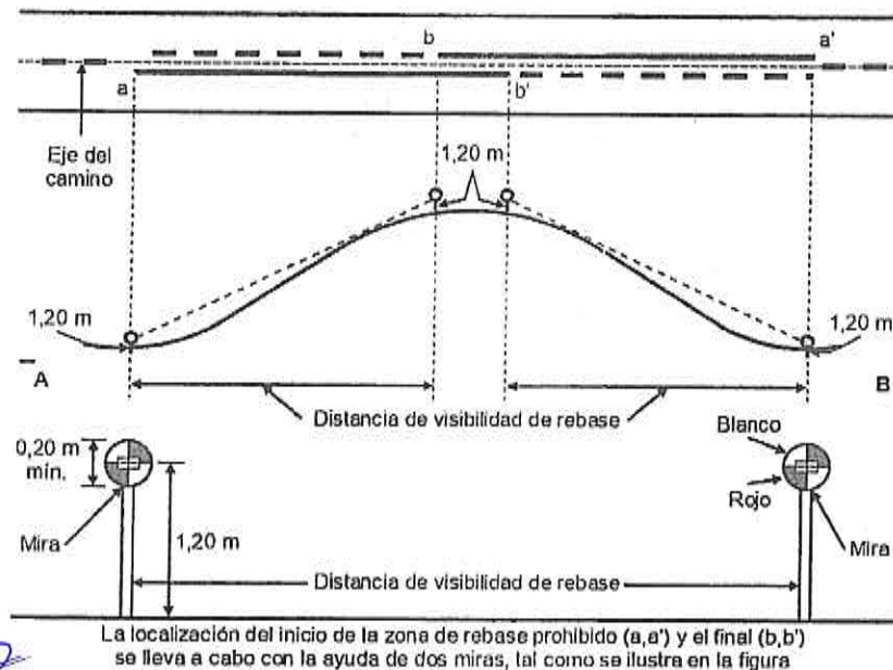
FIGURA 29.- Procedimiento para ubicar los límites de los tramos de rebase prohibido en curvas verticales
