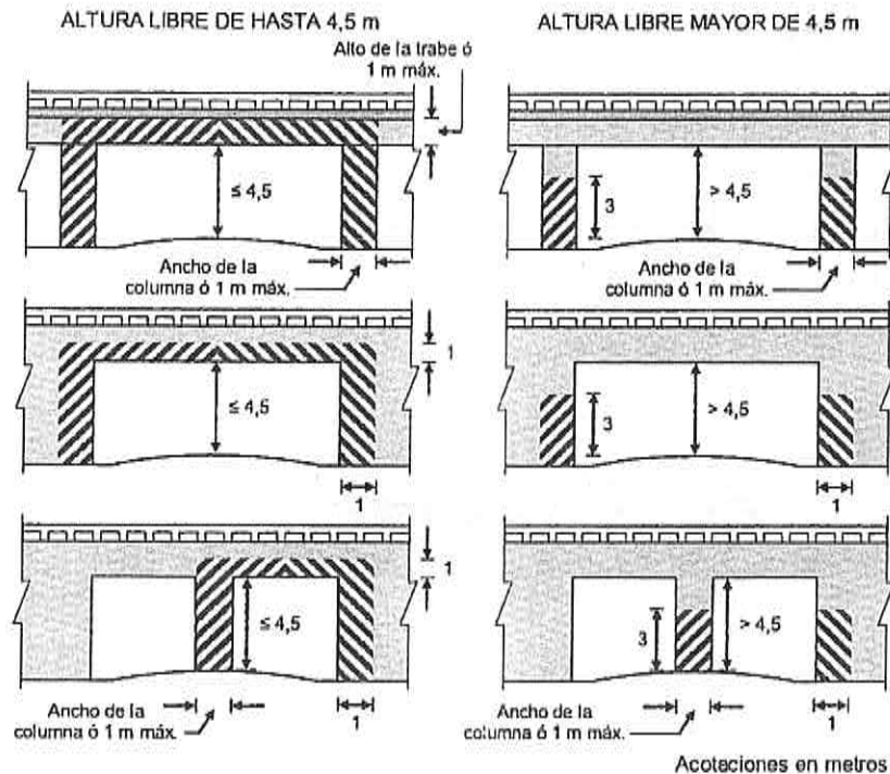
FIGURA 23.- Marcos en estructuras
