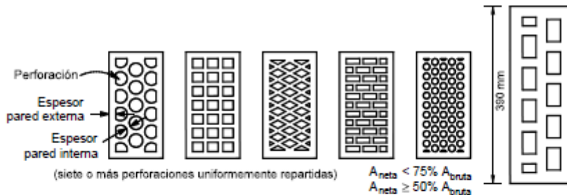
FIGURA 2.- Ejemplos de piezas multiperforadas
