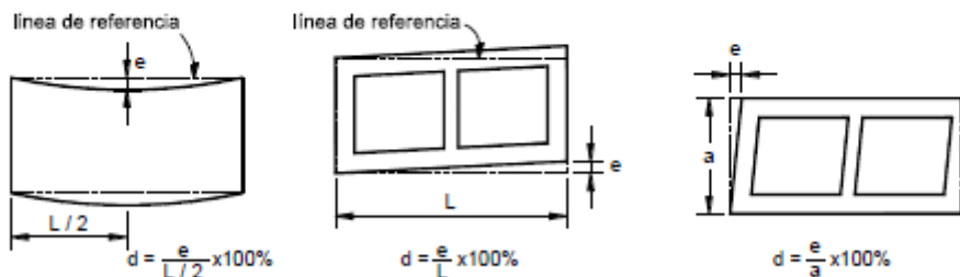
FIGURA 5.- Tolerancia de forma
