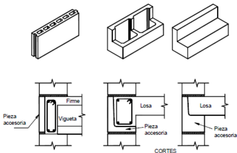
FIGURA 8.- Ejemplos de piezas especiales para rematar el borde de losas macizas o de vigueta y bovedilla con o sin dadas de borde
