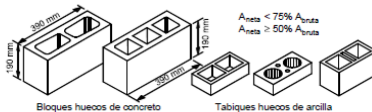
FIGURA 4.- Tipos comunes de piezas huecas
