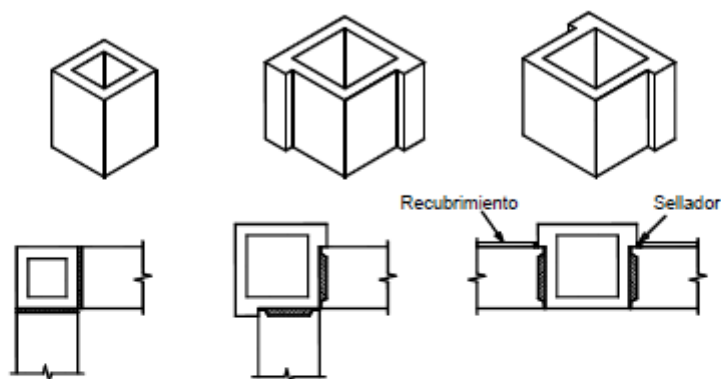
FIGURA 6.- Piezas para castillo
